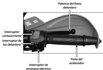
Imagen 1. Mando derecho.
