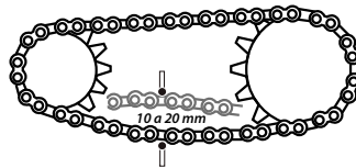
Imagen 29. Holgura de la cadena.
