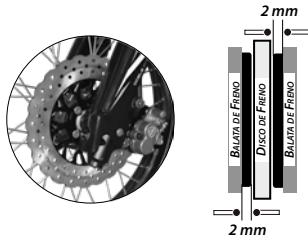
Imagen 24. Desgaste del freno delantero.
