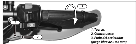
Imagen 21. Ajuste del puño del acelerador.
