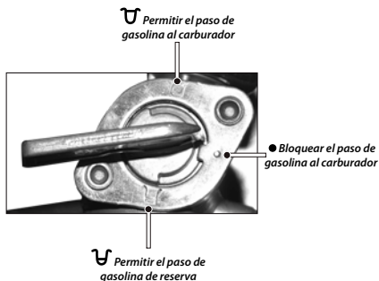
Imagen 12. Válvula de combustible.
