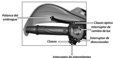
Imagen 4. Mando izquierdo.
