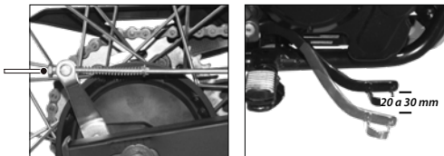
Imagen 26. Ajuste del pedal del freno trasero.
