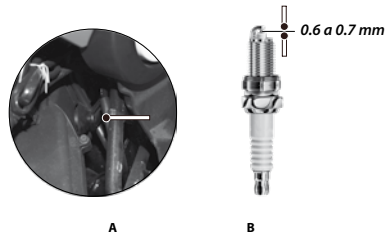
Imagen 15. Bujía.
